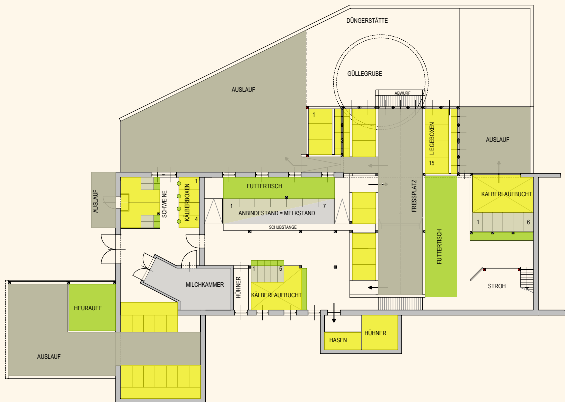
Grundriss – nach der Baumaßnahme
