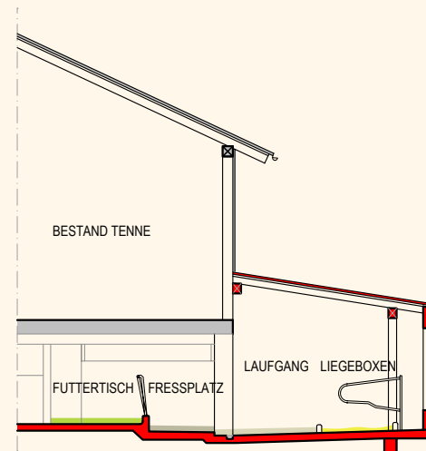
Schnitt – nach der Baumaßnahme
