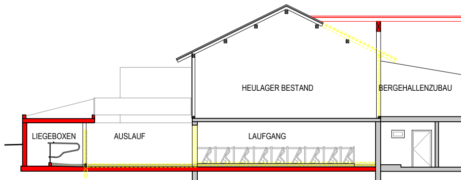
Schnitte – nach der Baumaßnahme
