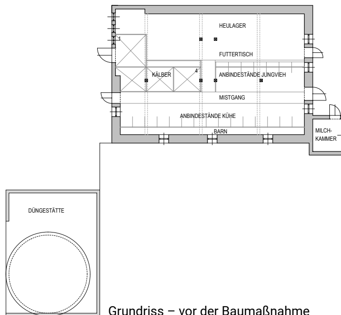
Grundriss – vor der Baumaßnahme
