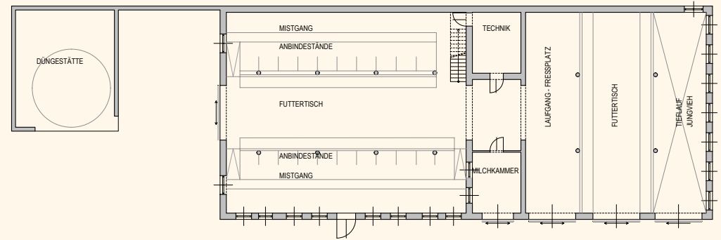
Grundriss – vor der Baumaßnahme
