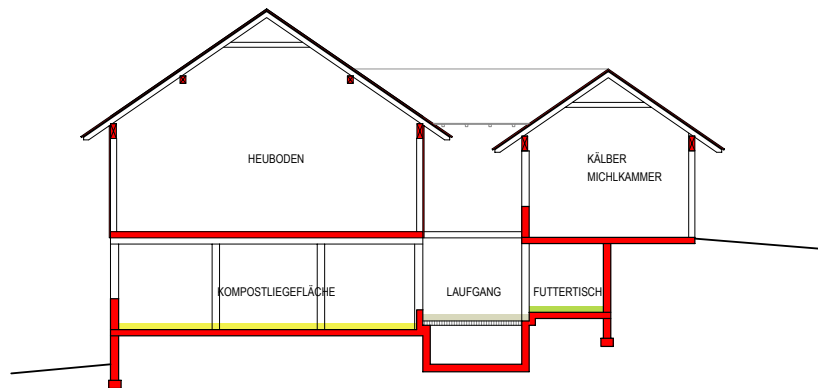
Schnitt – nach der Baumaßnahme
