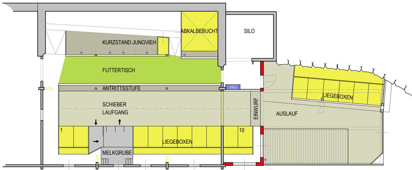
Grundriss – nach der Baumaßnahme
