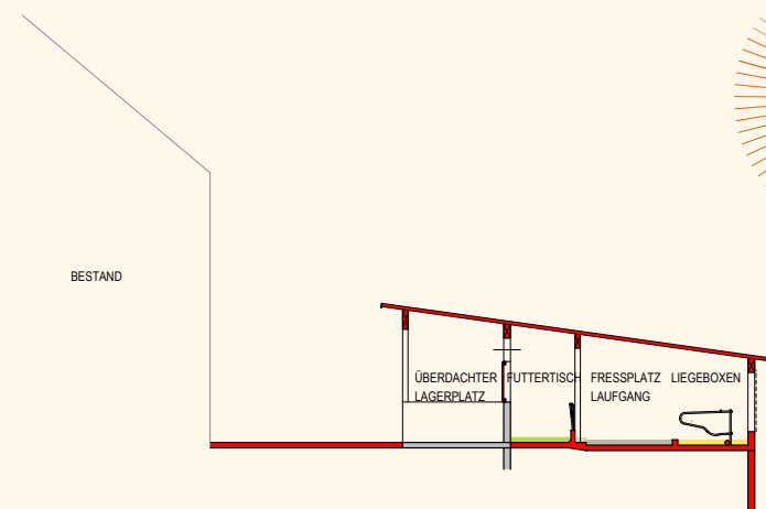
Schnitt – nach der Baumaßnahme
