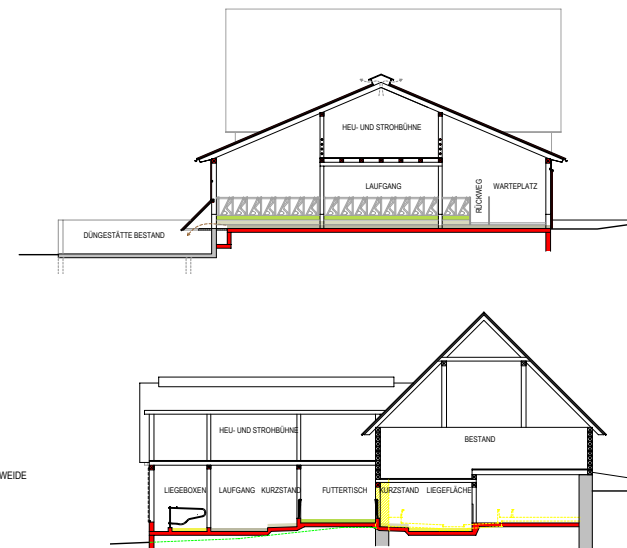
Schnitte der geplanten Baumaßnahme
