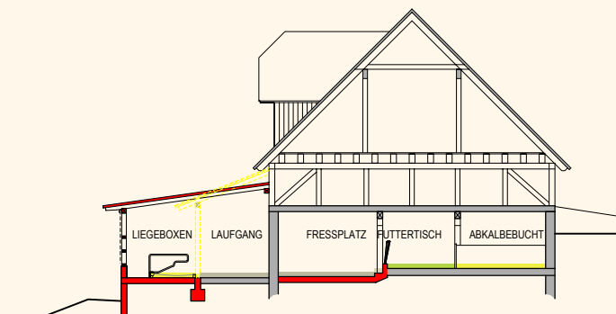
Schnitt – nach der Baumaßnahme
