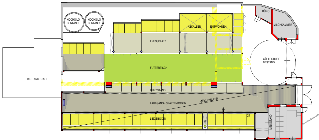
Grundriss – nach der Baumaßnahme
