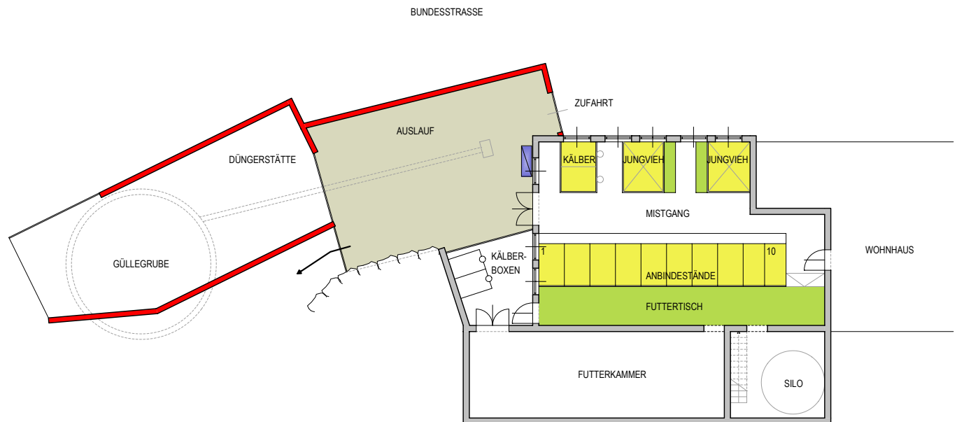
Grundriss – nach der Baumaßnahme
