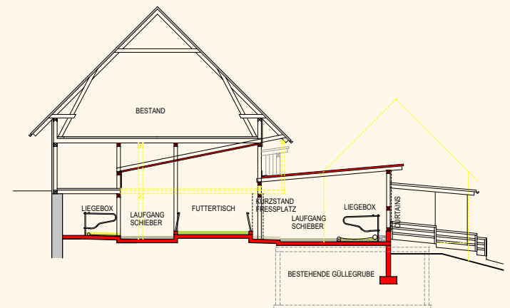
Schnitt – nach der Baumaßnahme
